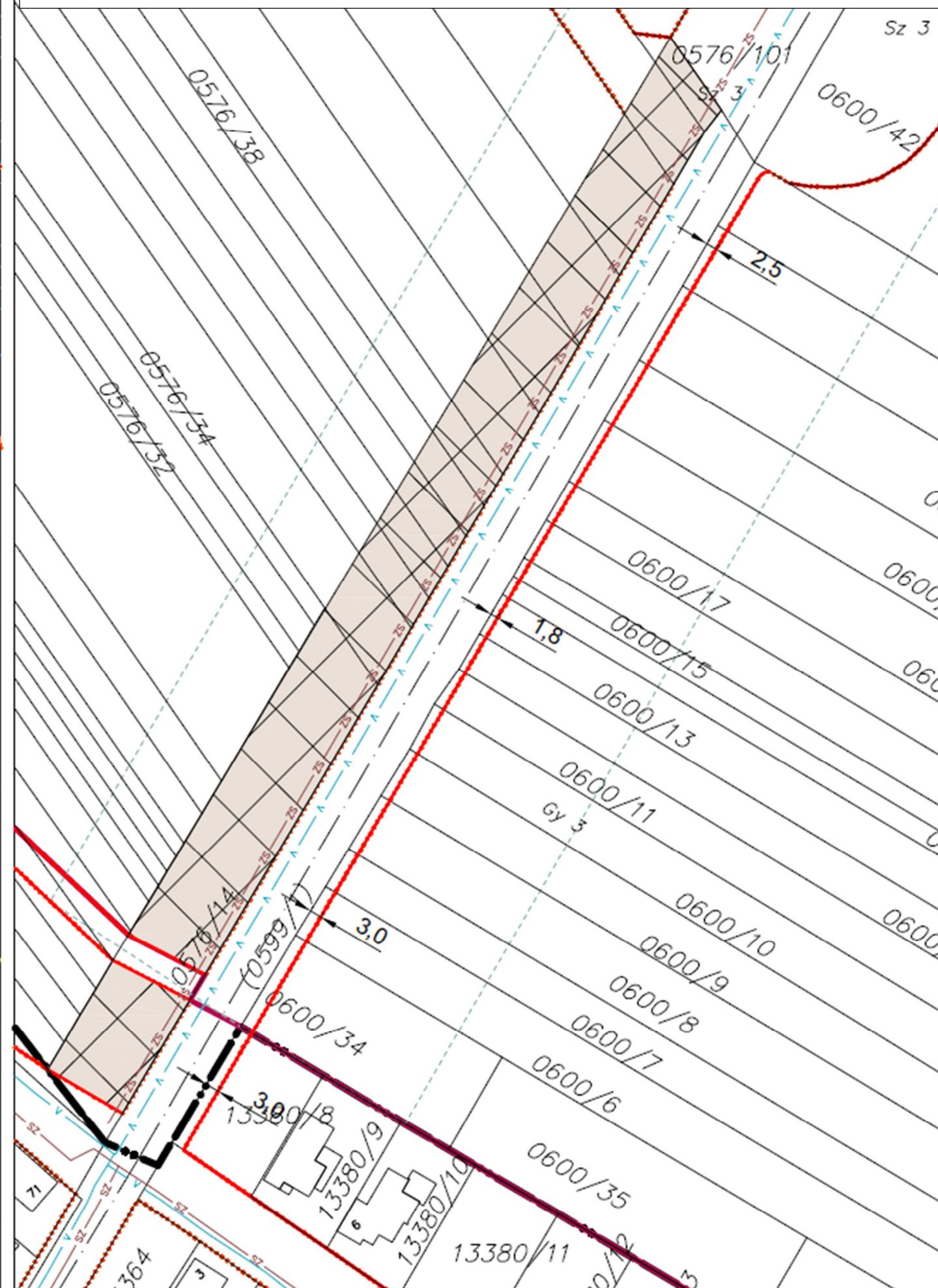
SZTM 2020-014 Győr - Bácsa, Bácsai út, szabályozási szélesség módosítása
